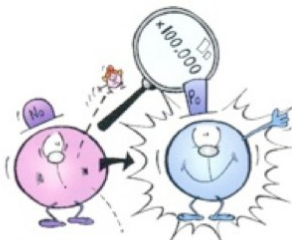
...produit par la transmutation d'un neutron en proton. Il y a aussi émission d'un neutrino, particule encore très mystérieuse.
